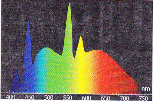
Profil spectral d'une lampe fluorescente dite « lumière du jour »
