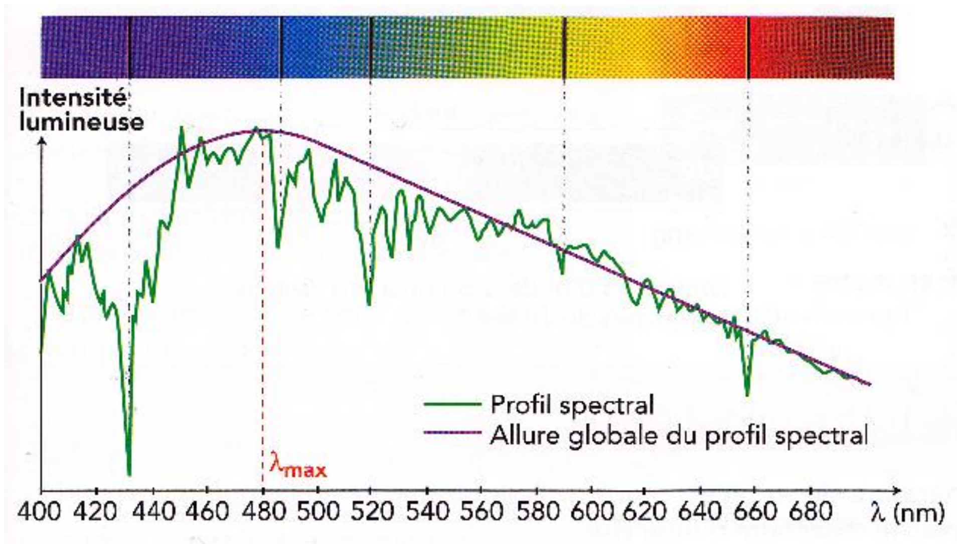
Profil spectral du Soleil
